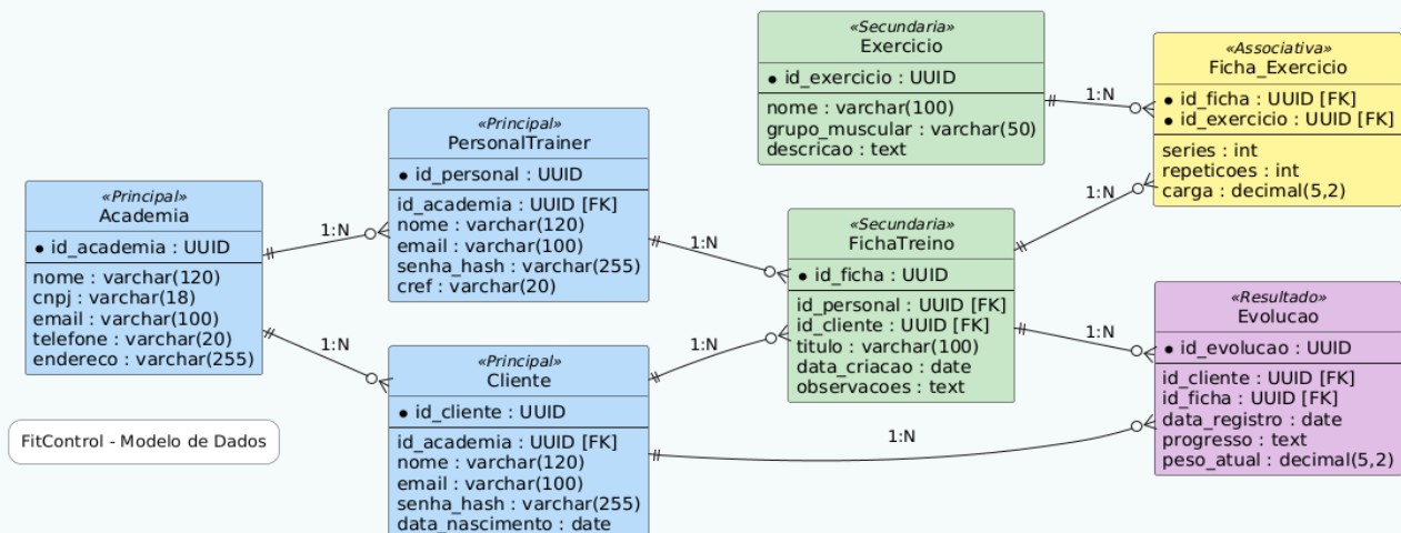
Modelo Entidade-Relacionamento - FitControl
